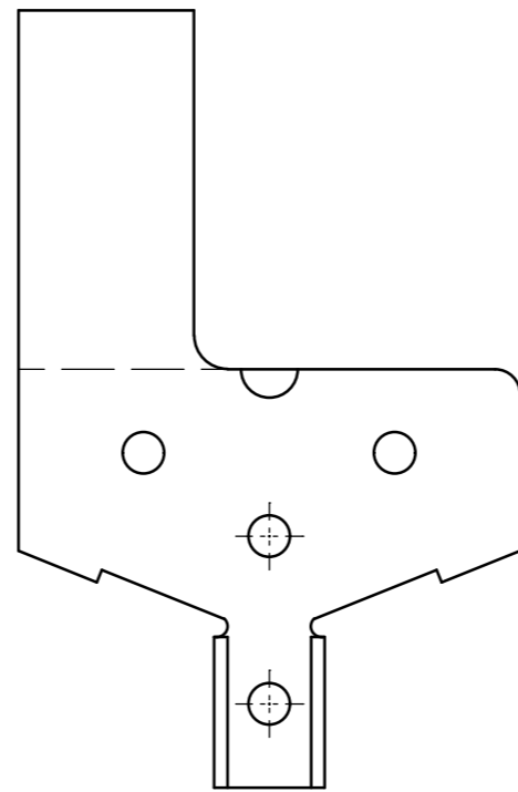
【背面図】
