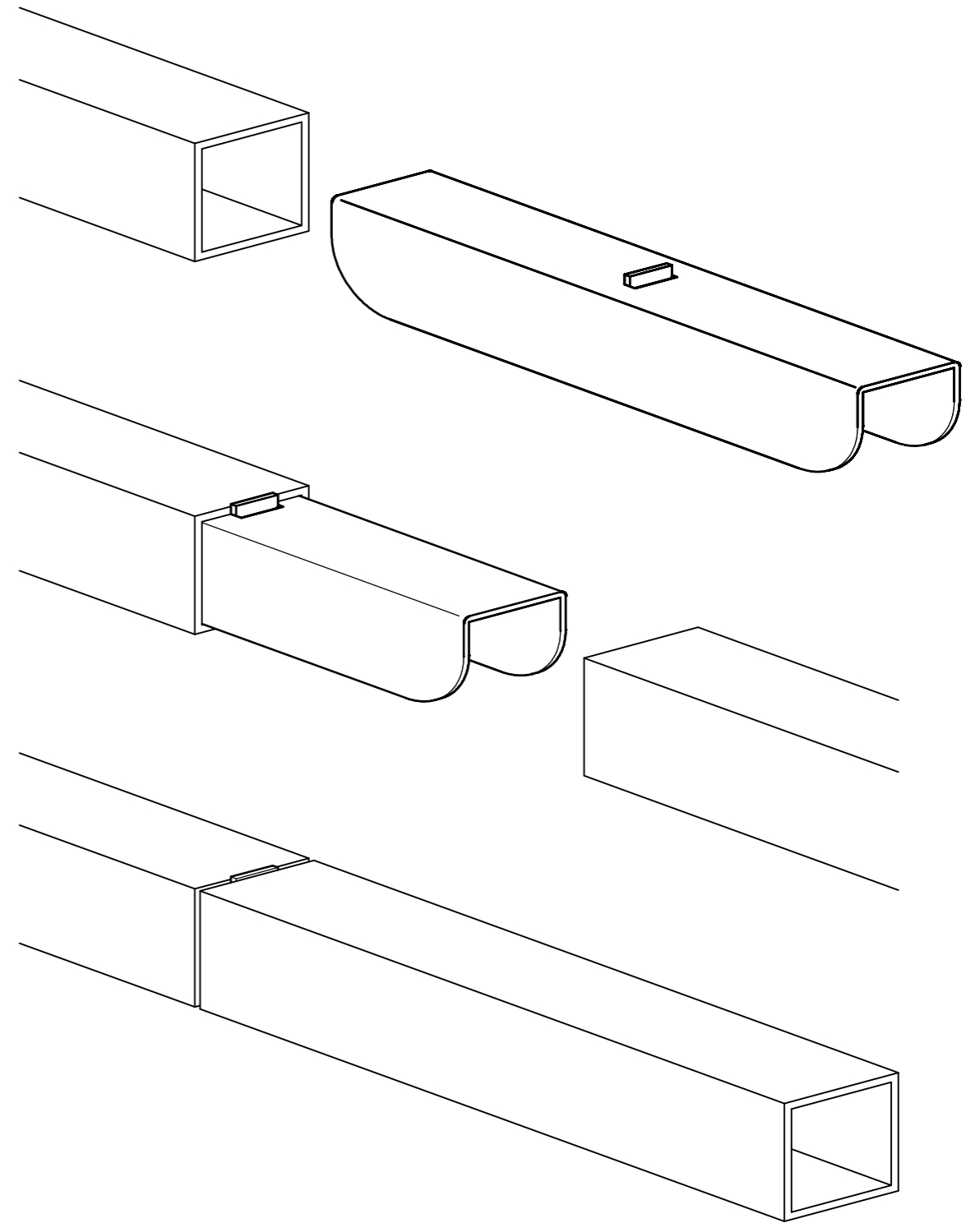
【取付図】
