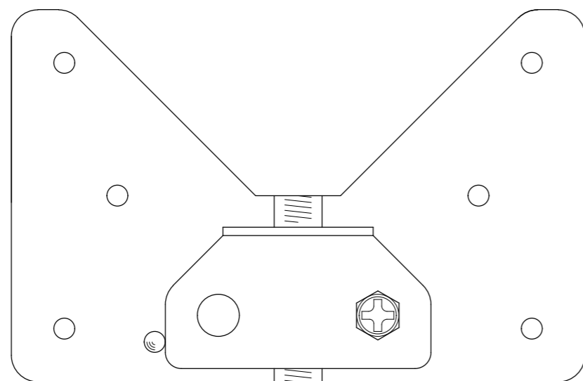
【正面図】
