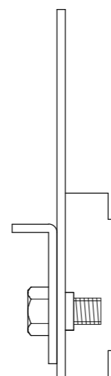
【右側面図】
