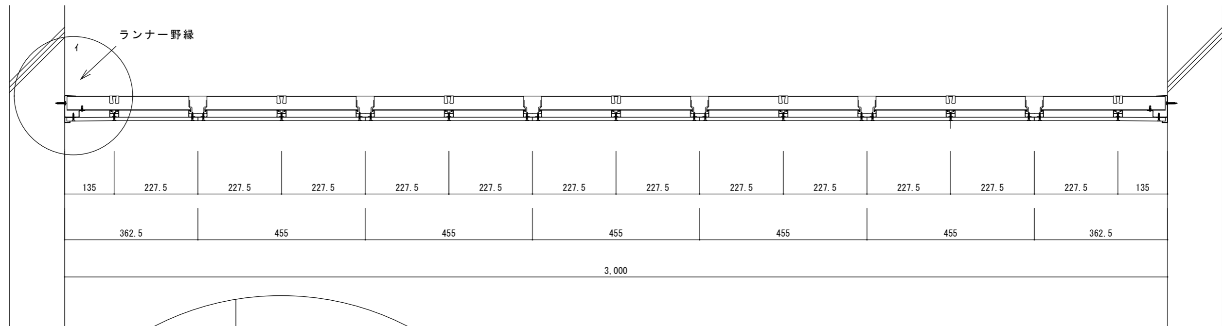
ライトゲージ天井 断面図 S=1/10
