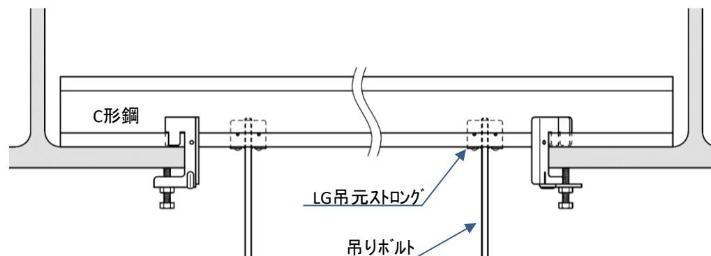
図8. H形鋼フランジの上にC形鋼を固定する場合
