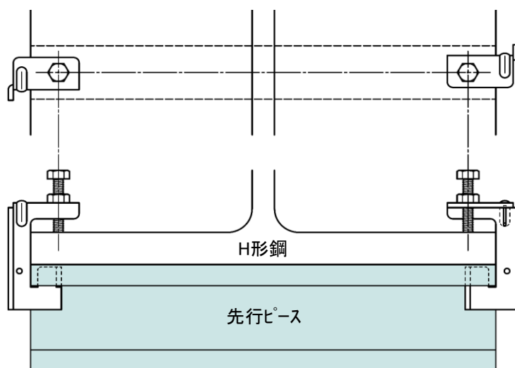
図6. H形鋼フランジ幅と先行ピースの長さが同じ場合
