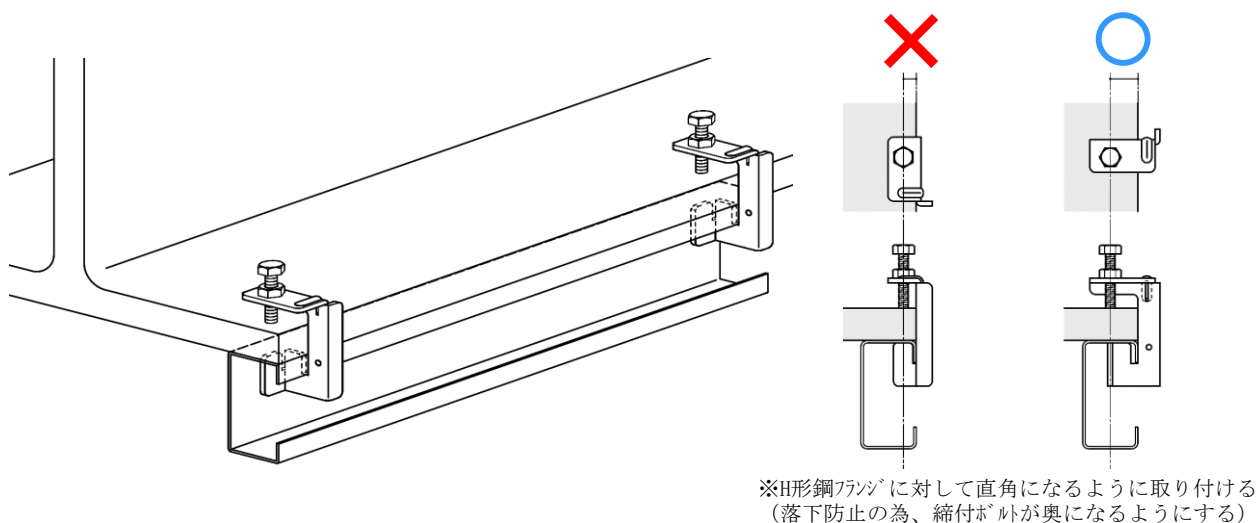
図7. H形鋼フランジに対して先行ピースが平行の場合
