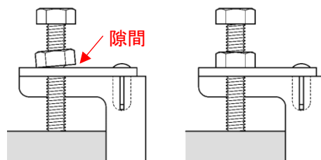
図5. ゆるみ止めナットの締付状態
